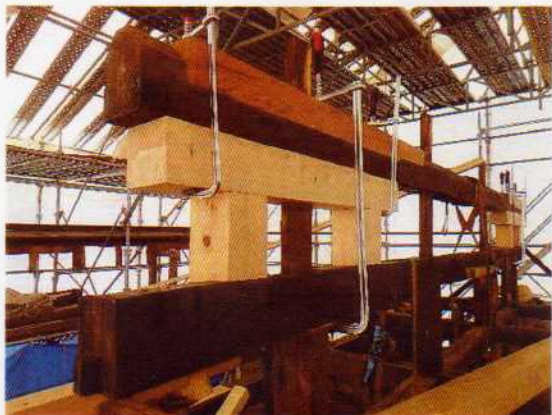
棟木補強組立 2018.5.16
